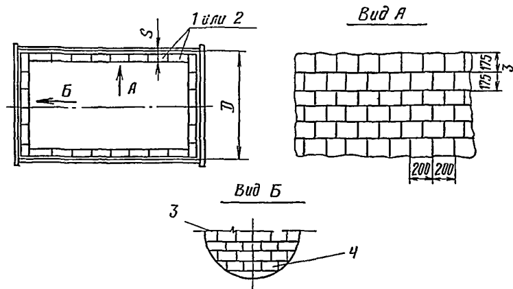
Рис.4. Схема футеровки габаритных горизонтальных цилиндрических аппаратов с плоскими днищами: 1 - плитка лекальная шпунтованная ПШШ; 2 - плитка лекальная ПЛ; 3 - плитка шпунтованная ПШ; 4 - плитка шпунтованная ПШ с подгонкой по месту
