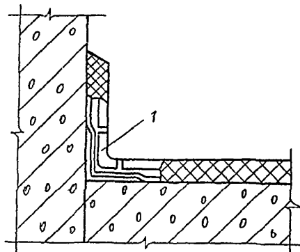
Рис.19. Схема облицовки плинтусов: 1 - плитка кислотоупорная керамическая угловая ПУ-1, спаренная угловая ПСУ-1,2
